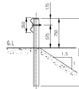
SIDE ELEVATION SCALE: NONE
