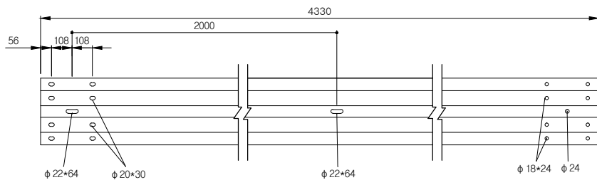
가드레일 SCALE: NONE
