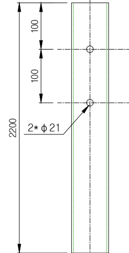
PIPE POST 상세도
