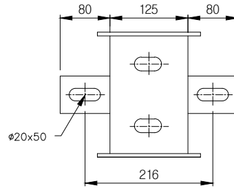
정면도
