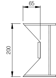
측면도
