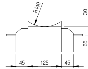
평면도
