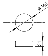
지주캡 상세도
