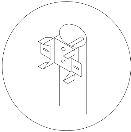
조립도 상세도
