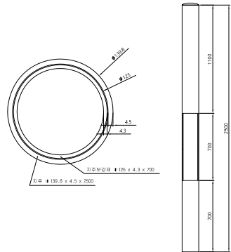
지주 상세도
