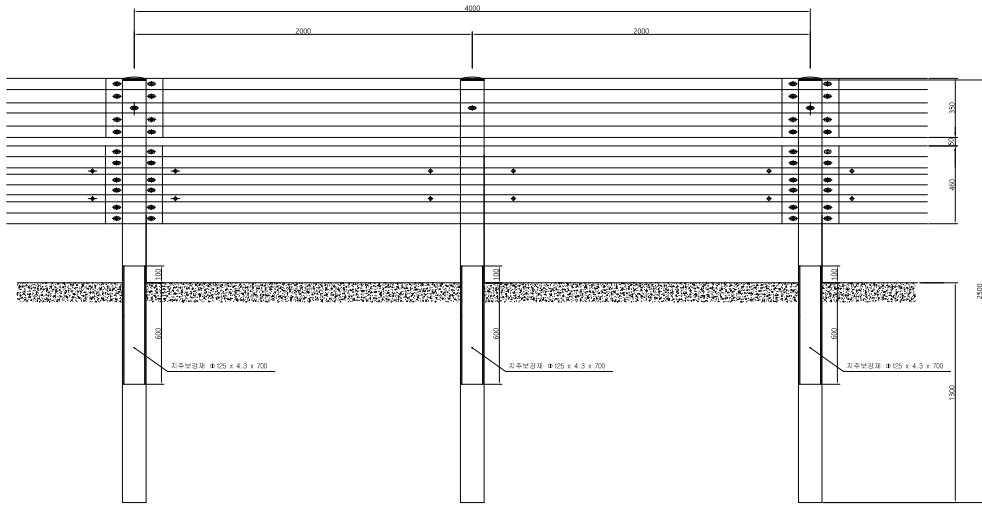
지주 상세도
