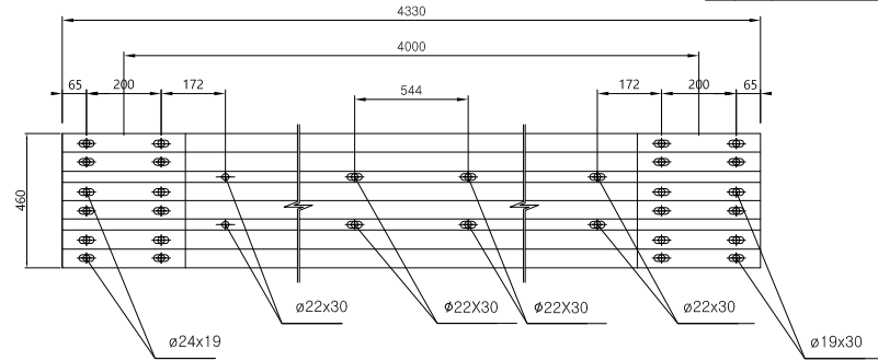
가드레일 상세도
