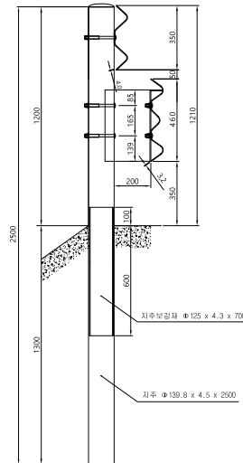
가드레일 설치도
