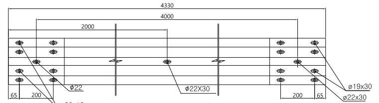
BOLT/NUT 상세도
