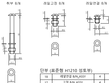
BOLT/NUT 상세도
