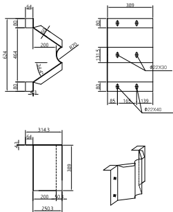
블럭아웃 상세도
