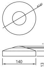
지주 덮개 상세도
