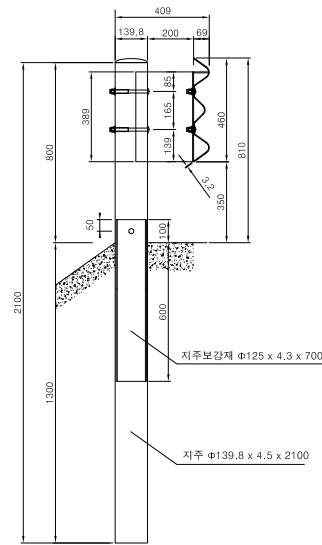
가드레일 설치도
