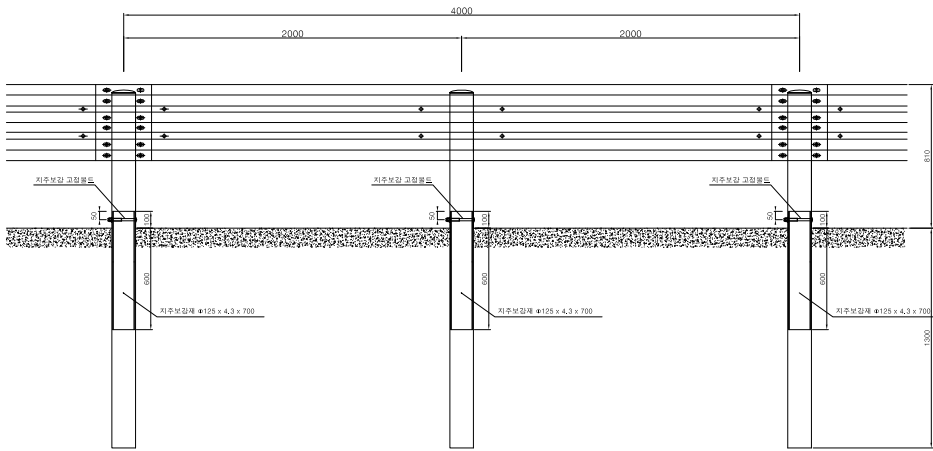
정면도
