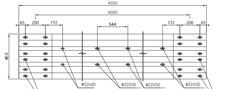
정면도
