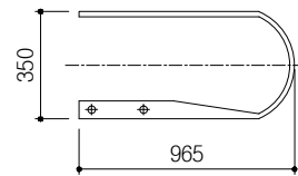
단부레일 상세도
