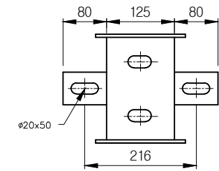
정면도
